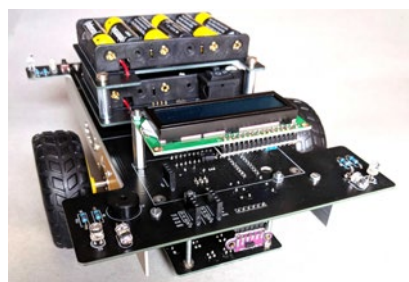
Selbstfahrender Roboter, selbst gebaut
