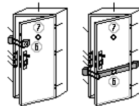
Aufbauschloss Panzerriegel
